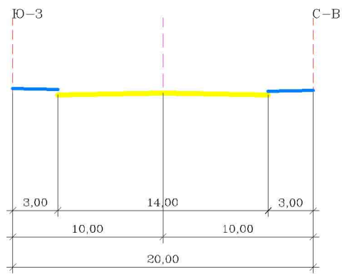
ПОПЕРЕЧНЫЙ ПРОФИЛЬ Магистраль городского значения участок от ул.Преображенского до ул.Ленинградской (до развязки)
